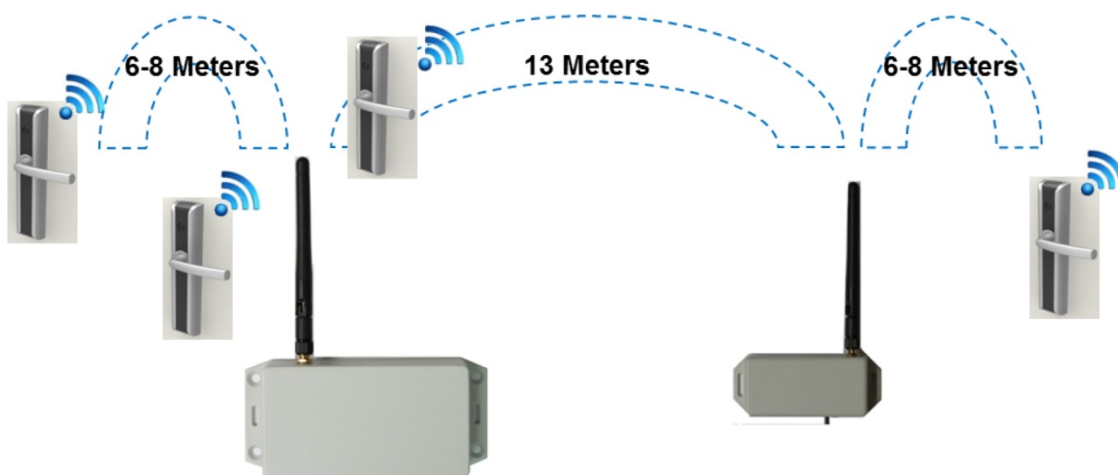
Σχήμα 4 – Gateway στο κέντρο και για επικοινωνία με αρκετές κλειδαριές και επιπλέον Repeater για επικοινωνία με απομακρυσμένη κλειδαριά.
