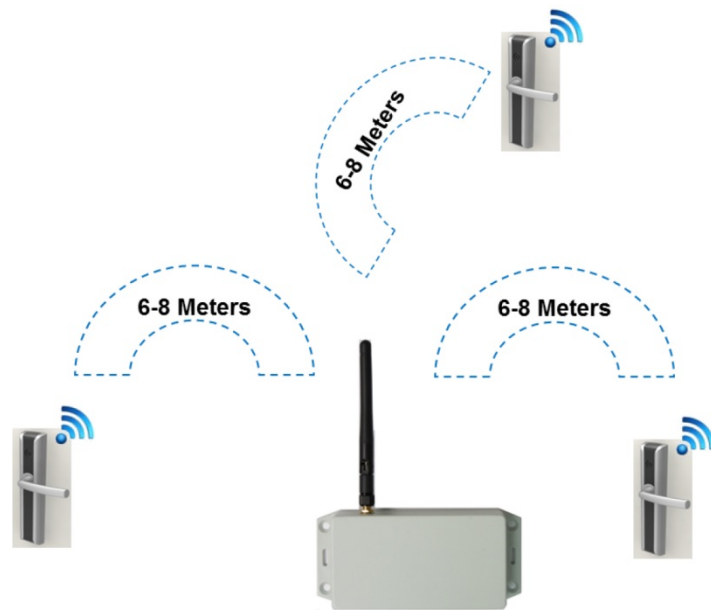
Σχήμα 1 – Gateway στο κέντρο και κλειδαριές σε κοντινή απόσταση γύρω του
