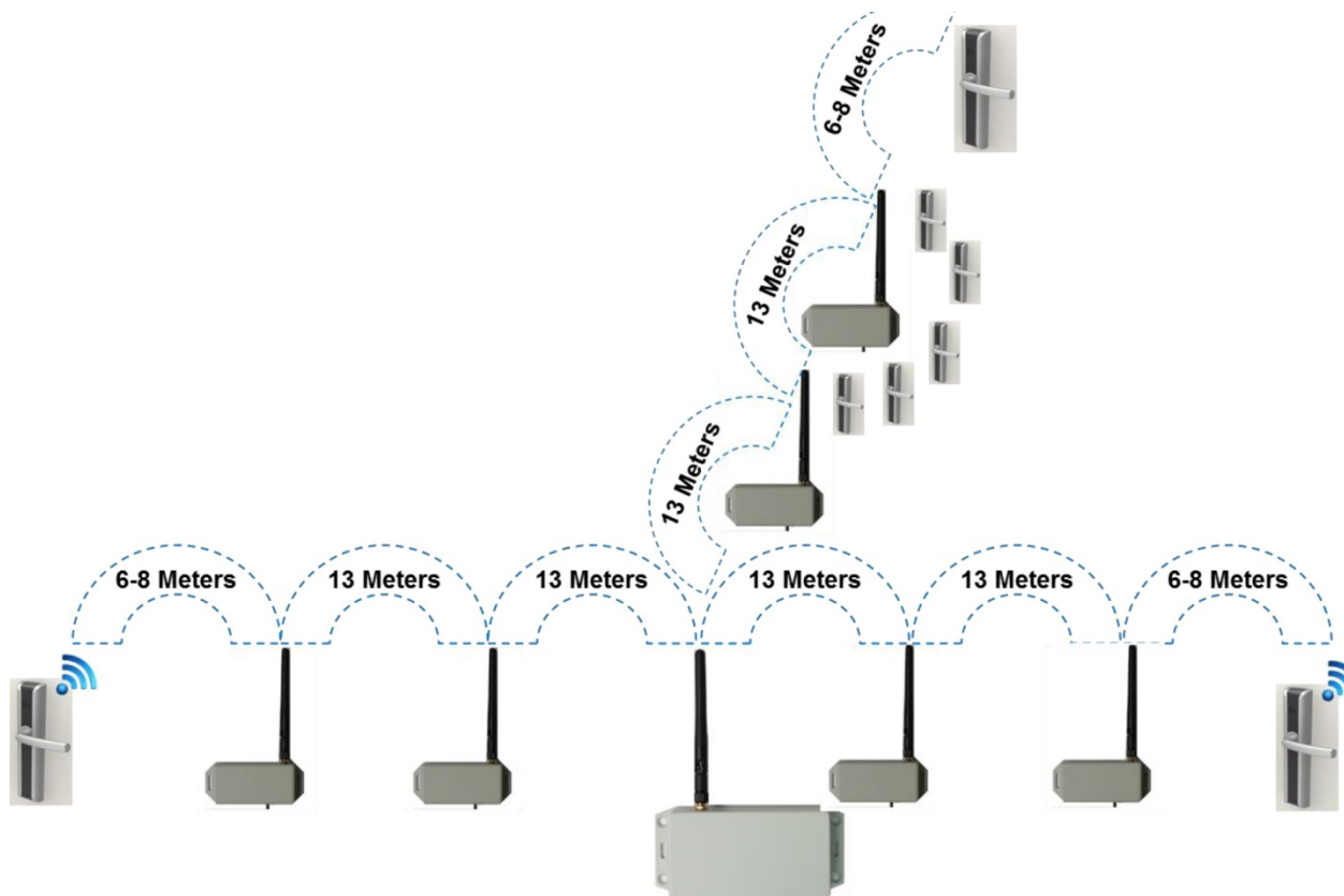
Σχήμα 3 – Gateway στο κέντρο και διάφοροι Repeaters για επικοινωνία με περισσότερες κλειδαριές.
