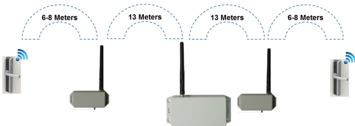
Σχήμα 2 – Gateway στο κέντρο, repeaters σε κάθε πλευρά για επικοινωνία με κλειδαριές σε μακρινή απόσταση
